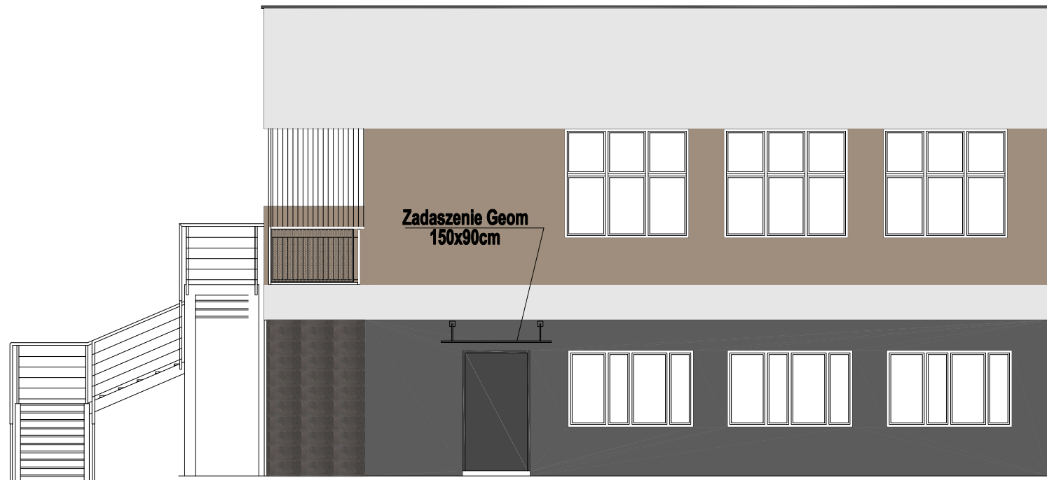
ELEWACJA POŁUDNIOWA
